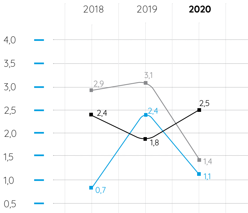
Concentrazioni rilevate \text{NO}_2 | figura 11
