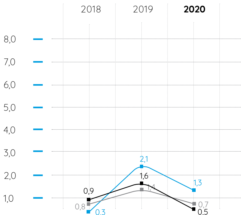
Concentrazioni rilevate \text{NO} | figura 12
