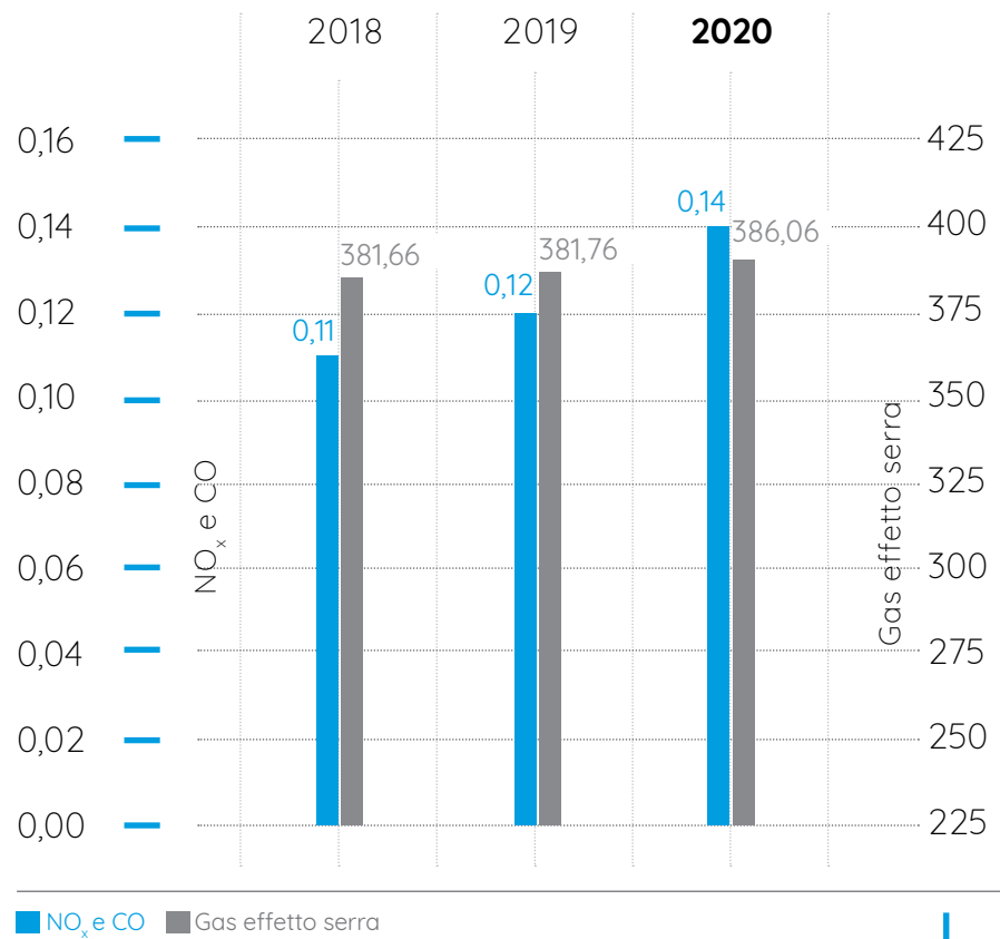
Emissioni specifiche settoriali | figura 10
